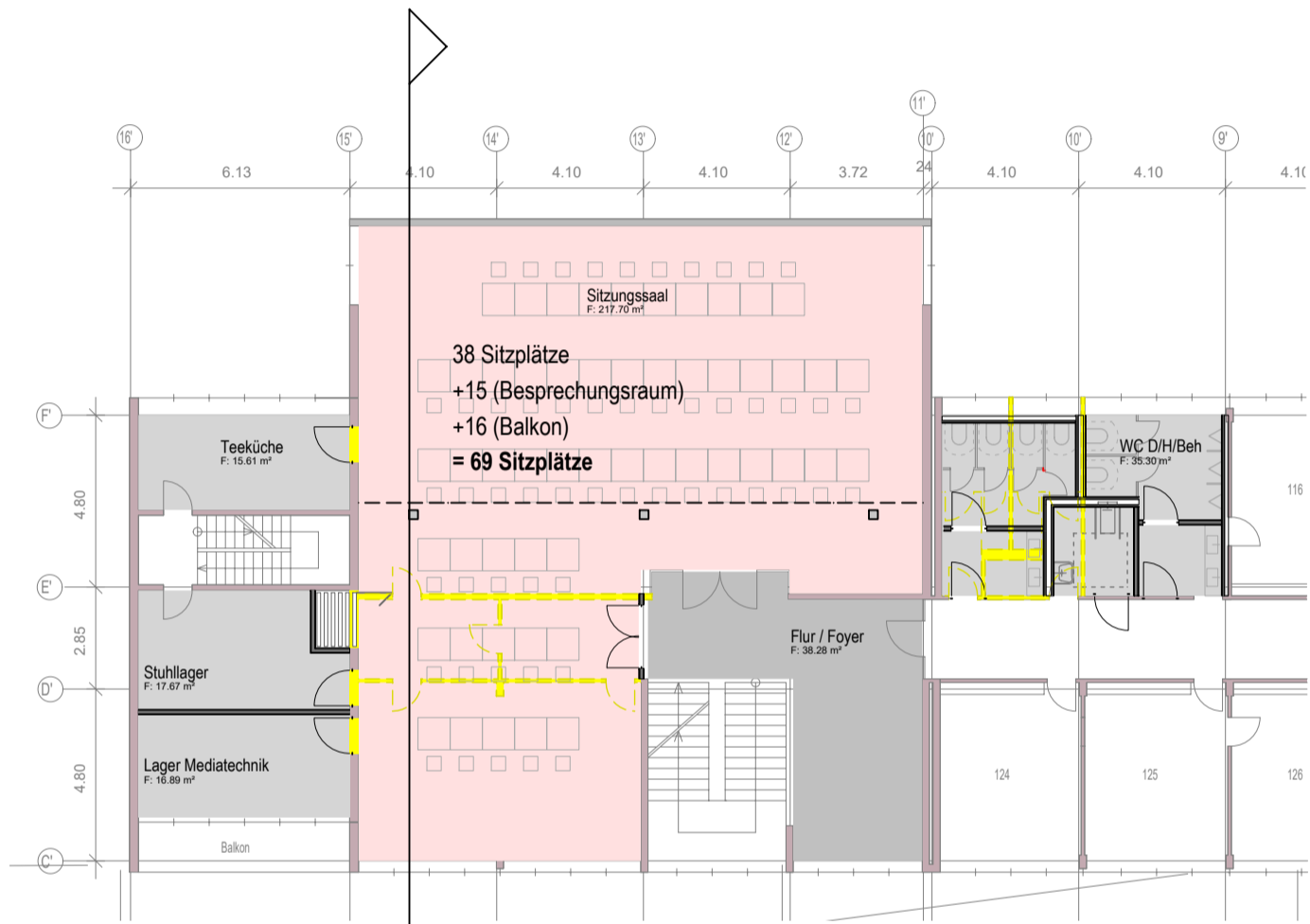
Grundriss 2.OG
